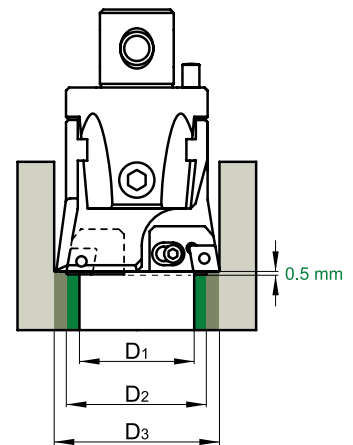
Ступенчатое растачивание
