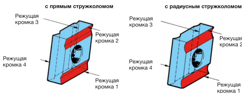
Двусторонние режущие пластины с прямым стружколомом (рис.5) обеспечивают образование короткой стружки, обязательной при многолезвийной обработке. Геометрия пластины с 4 режущими кромками уменьшает стоимость одной кромки.
