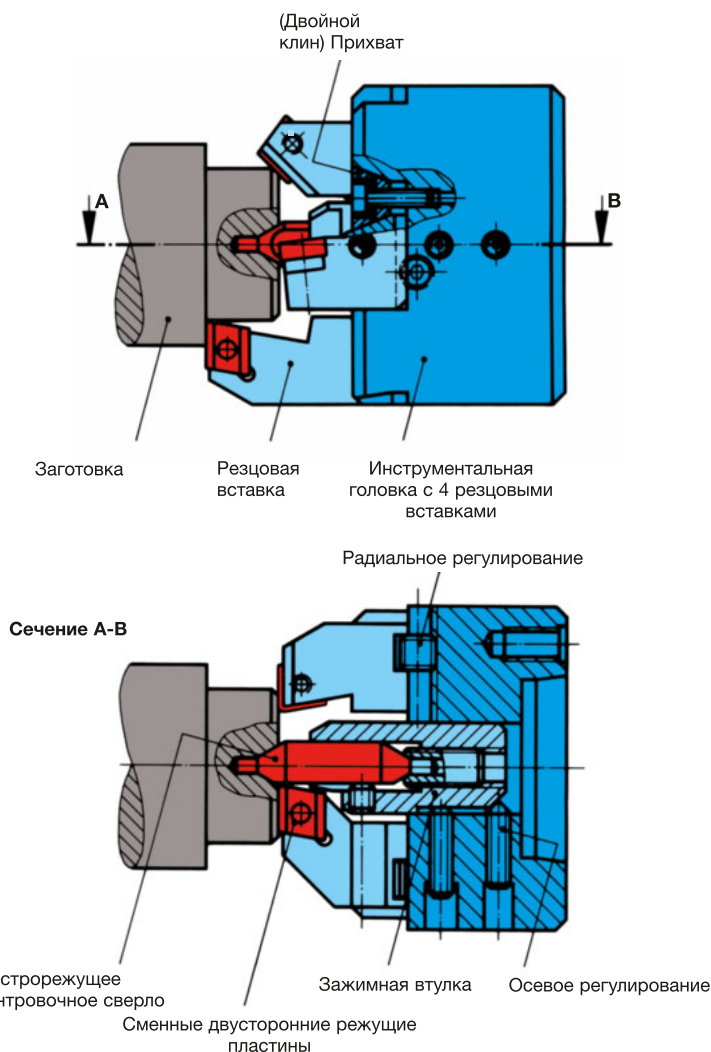
Рис. 4: Возможно крепление инструментальной головки на базовые оправки всех известных исполнений шпинделей станков и быстросменных систем. Посредством замены резцовых вставок и зажимной втулки одна и та же инструментальная головка быстро переналаживается под самые различные задачи по обработке. Пакет тарельчатых пружин зажимает резцовые вставки клиновым прихватом.
