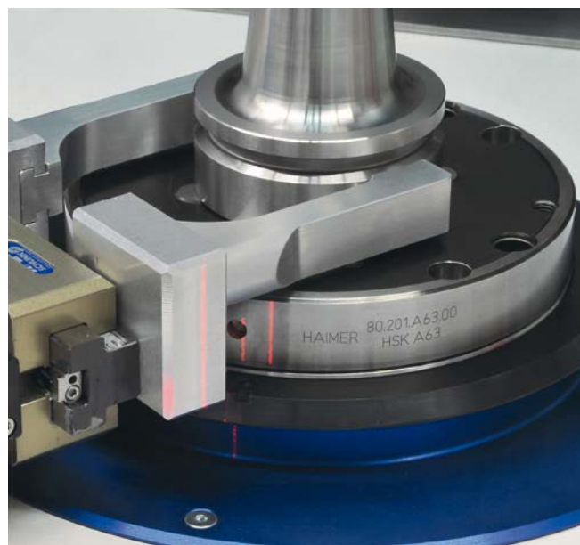
Интегрированный адаптер для балансировки и захват для автоматического измерения индексированием. Integrated adapter for balancing and gripper for automatic measurement with indexing.
