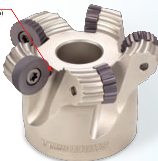
Рис. 8. Круглая пластина с гладкой режущей кромкой, установленная для улучшения параметров шероховатости поверхности обработки
