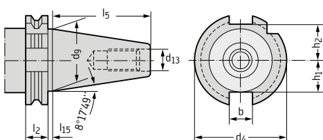
Базовый держатель (СК) DIN 69 871, часть 1, форма А
