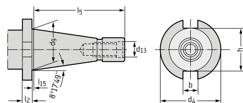
Базовый держатель (СК) DIN 2080
