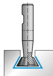
Фрезы для пазов типа ласточкин хвост
