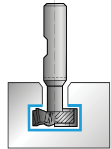
Фрезы для Т-образных пазов
