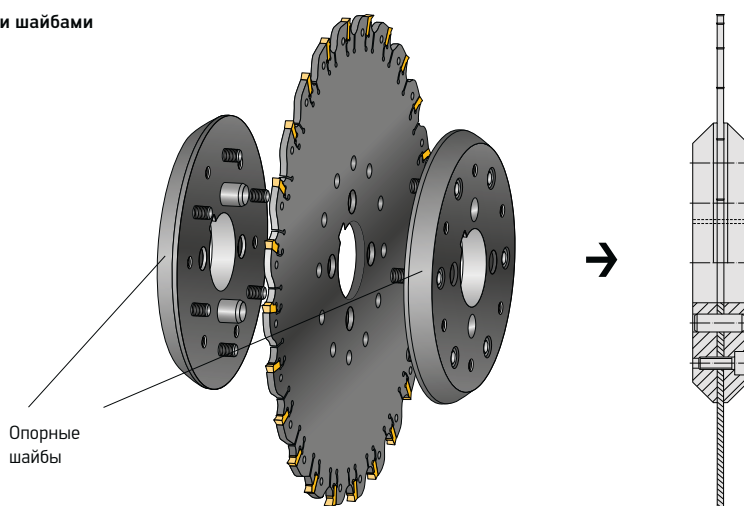
Сборка с опорными шайбами
