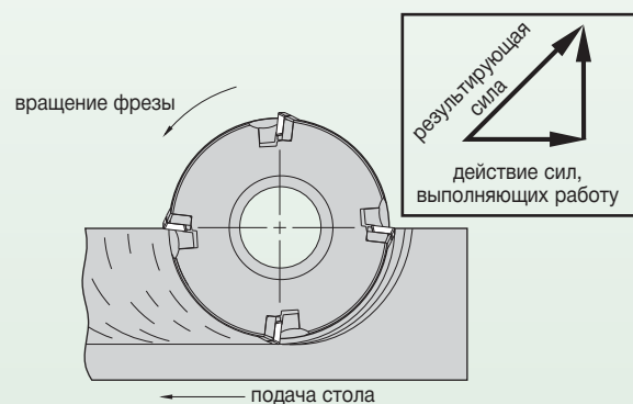
Встречное фрезерование
