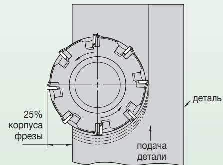
Положение фрезы
